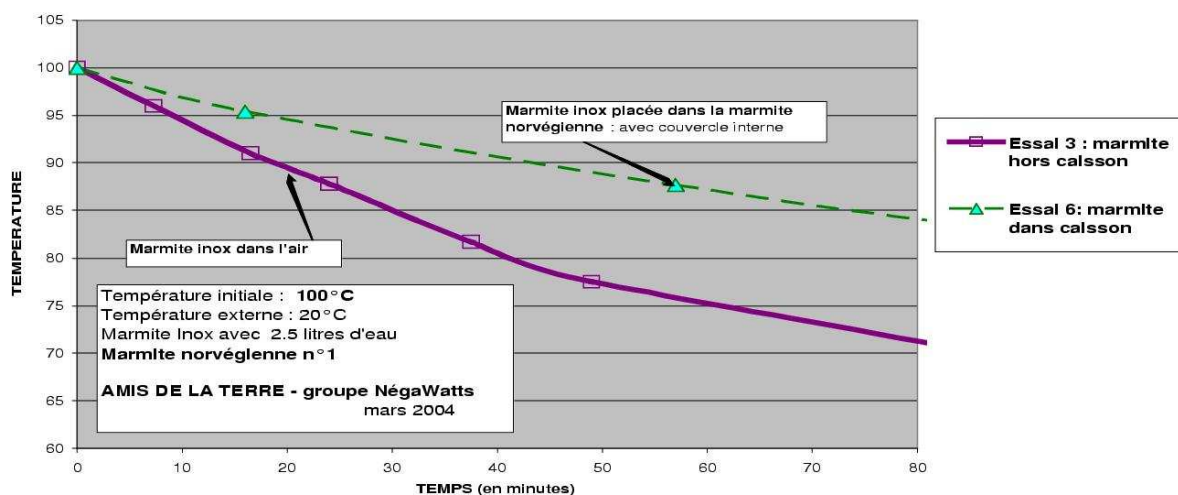
PERTE DE TEMPERATURE - TEST MARMITE NORVÉGIENNE : mars 2004
